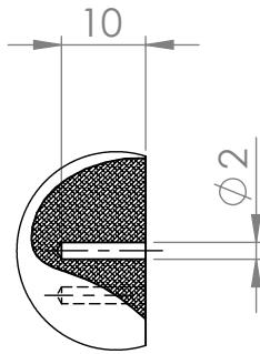
DETAY A ÖLÇEK 1 : 1
